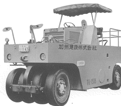
タイヤローラー
